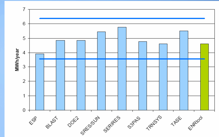
Ψυκτικά φορτία
